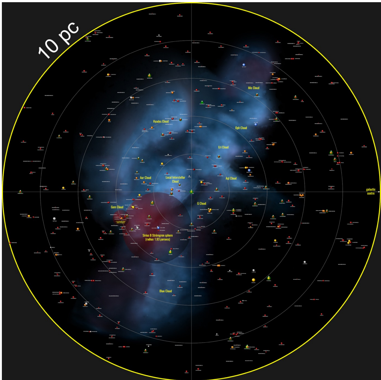
Vista proyectada desde arriba del plano galáctico. Los círculos concéntricos están separados 2 parsecs. Los círculos verdes alrededor de las estrellas indican el número de exoplanetas confirmados. Créditos galaxymap.org, Twitter: @galaxy_map
